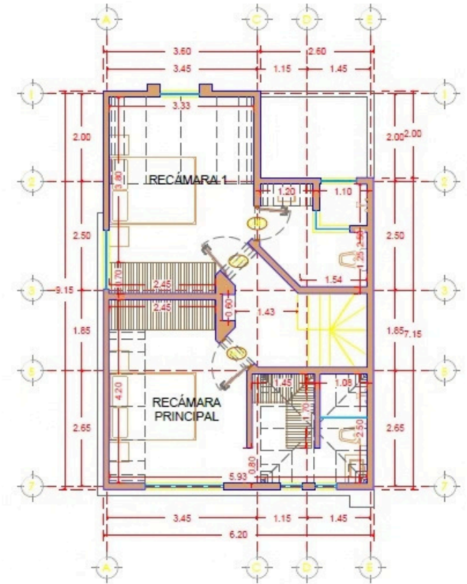
PLANTA ALTA
