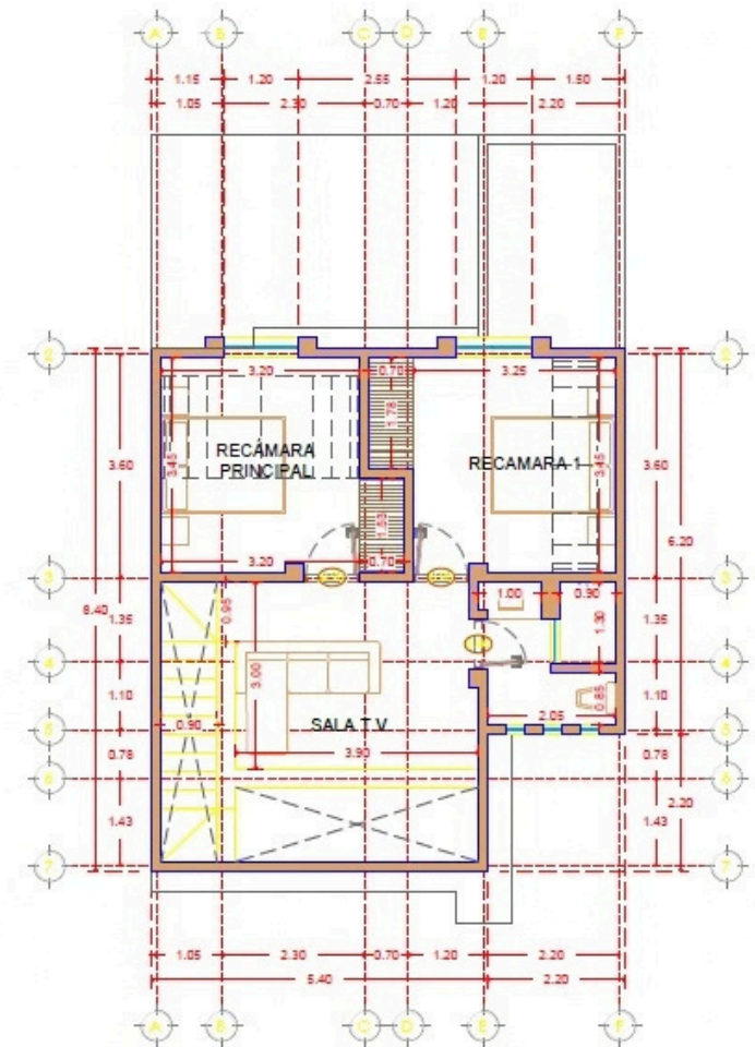
PLANTA ALTA
