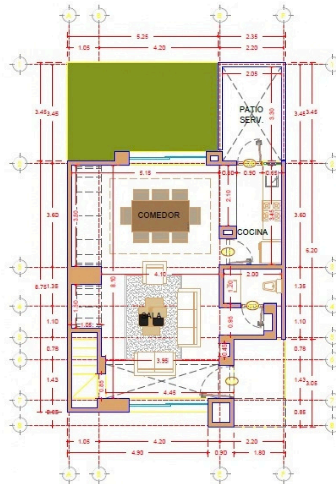
PLANTA BAJA
